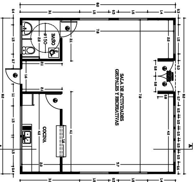
PLANTA TERCERO
